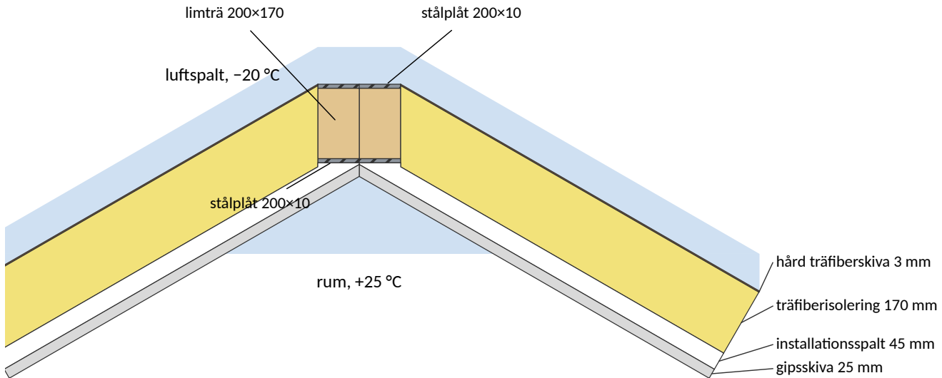
Figur 1: Tvärsnitt genomnocken. Modellen omfattar 1 000 mm tak, mätt längs takfallet, på var sida om balken. Taket har takvinkeln 30°. Isoleringens ovansida ligger i balkens överkant. Under isoleringen finns en installationsspalt med glespanel och därunder gipsskivan, vars topp ligger strax under balkens underplåt.
