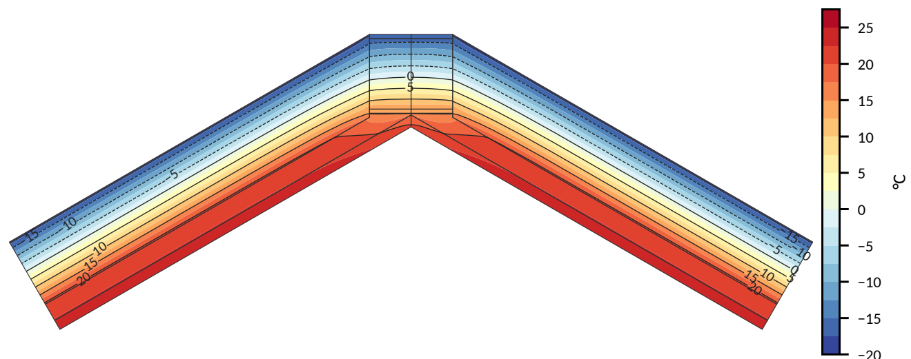
Figur 2: Temperaturfält, grundfallet. Ute -20 °C i luftspalten, inne +25 °C.
