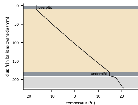
Figur 4: Temperatur längs nockens mitt.
